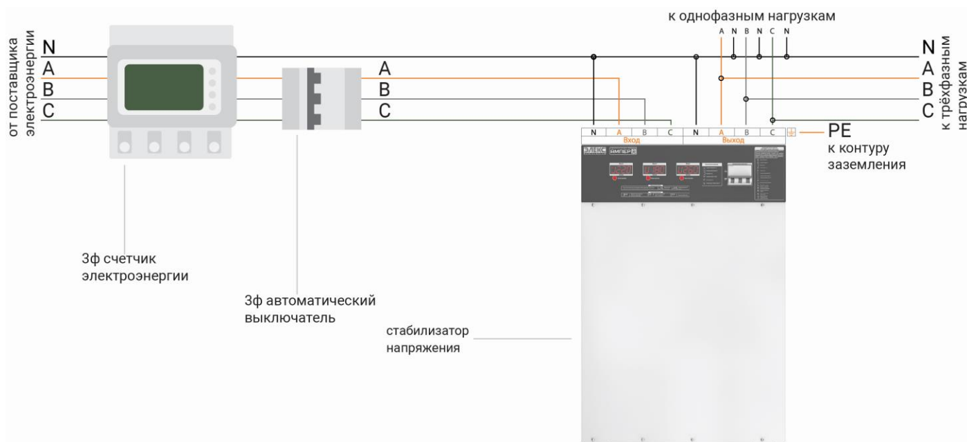
Рисунок 6. Схема подключения стабилизатора к трёхфазной сети
