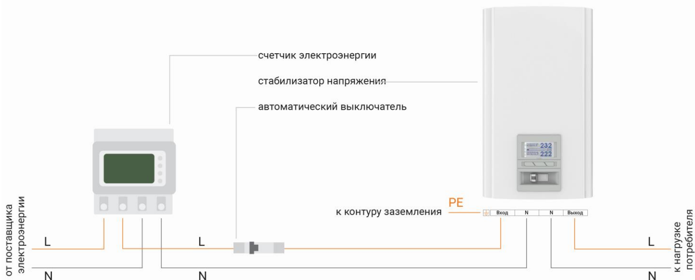
Рисунок 10. Схема подключения Герц и Герц-Дуо к однофазной сети
